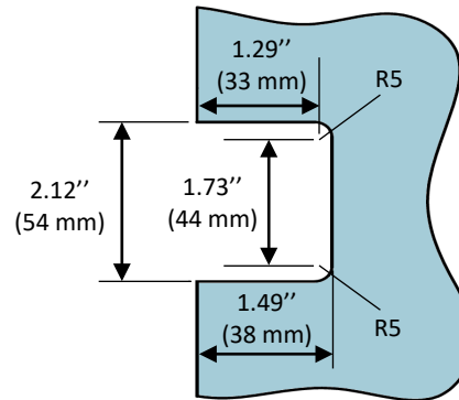
Gabarit pour gâche sur le verre
