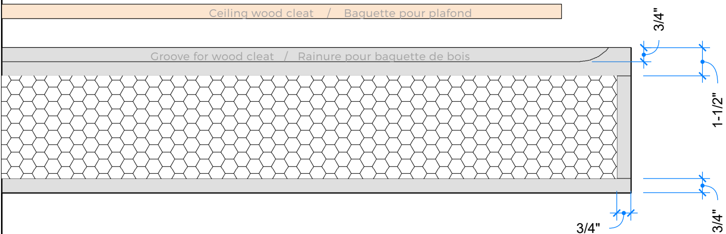
Internal details / Détails internes
